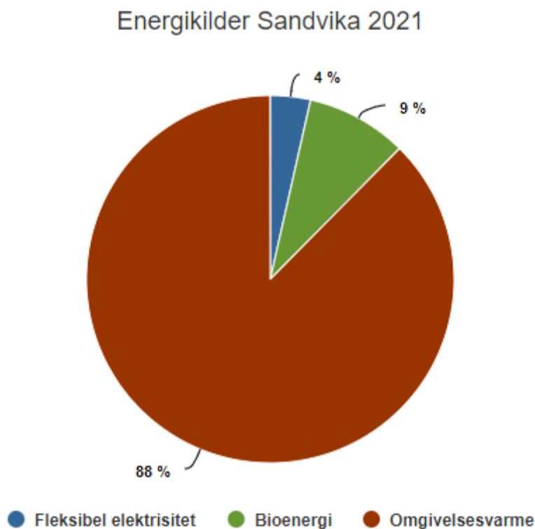
Figur 1 Energikilder Sandvika 2021
